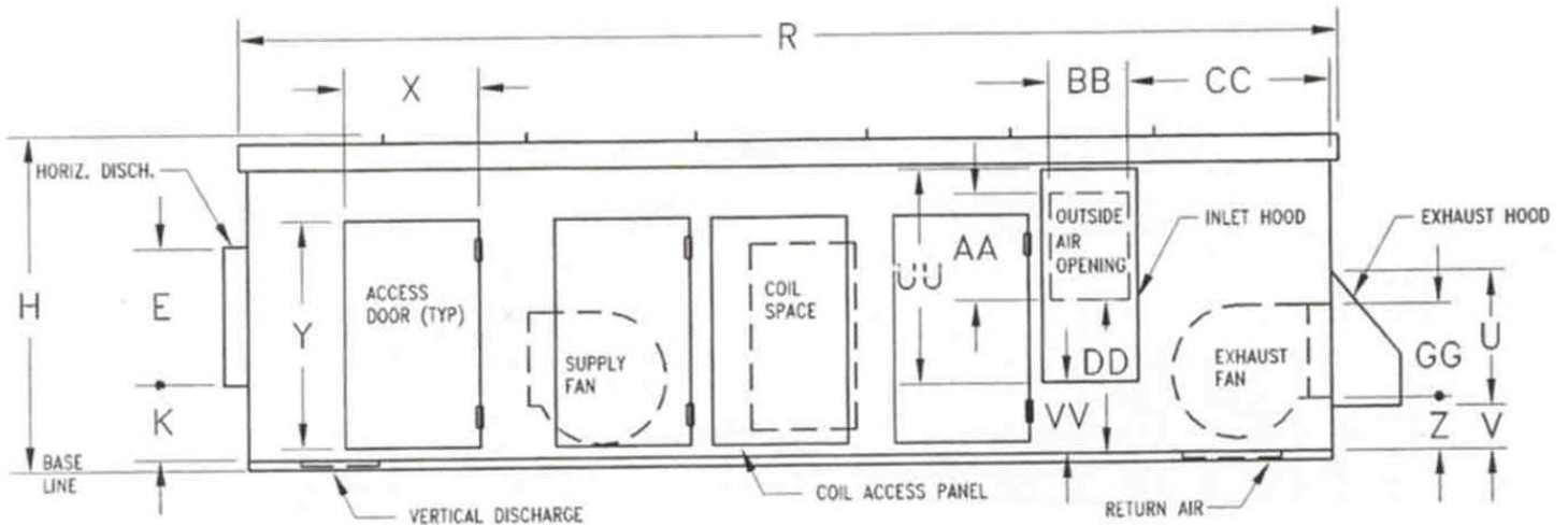
ELEVATION
